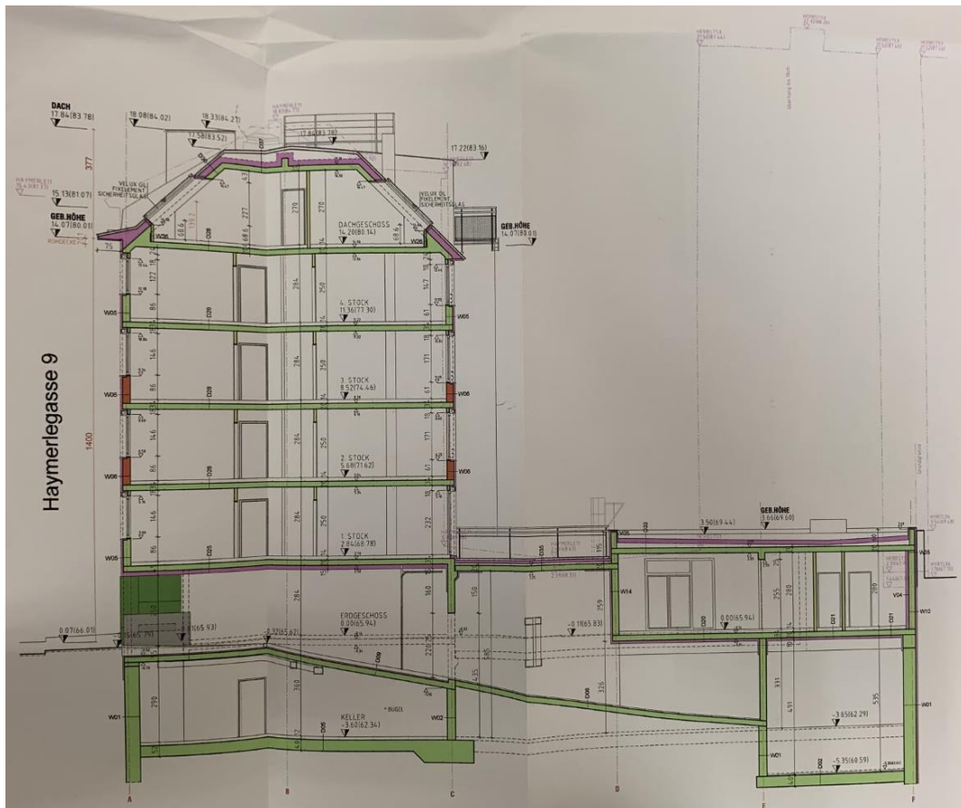
Schnitt A-A (Einreichplan Februar 2010)
