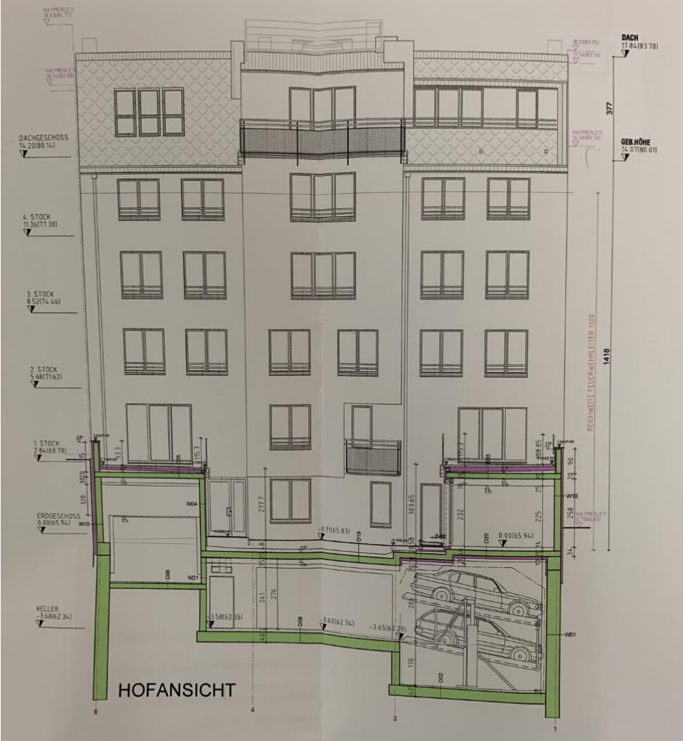
Hofanischt (Einreichplan Februar 2010)
