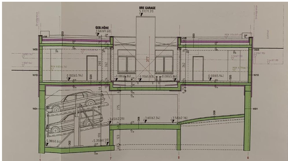
Schnitt C-C (Einreichplan Februar 2010)
