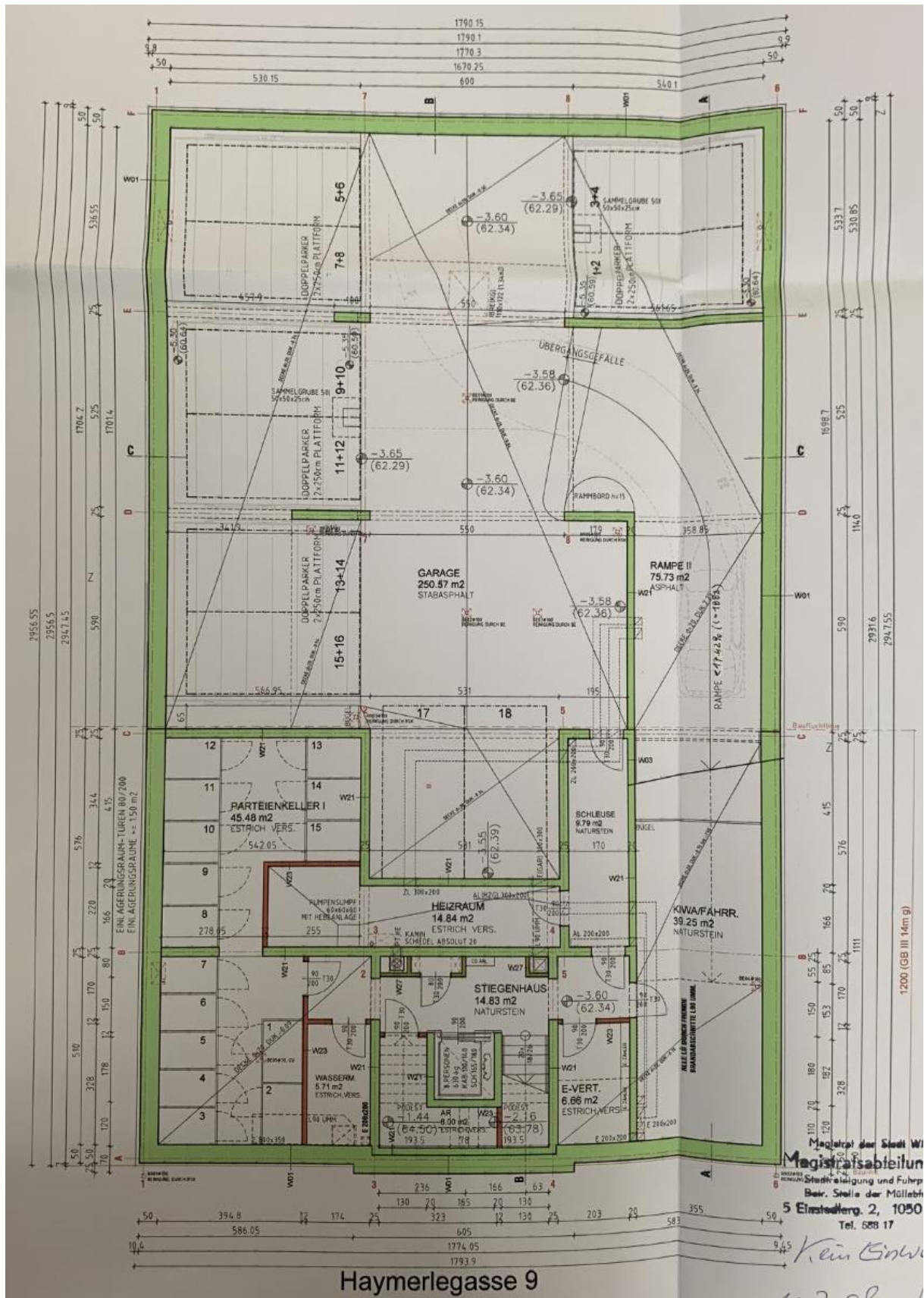
Grundriss Kellergeschoß (Einreichplan Februar 2010)
