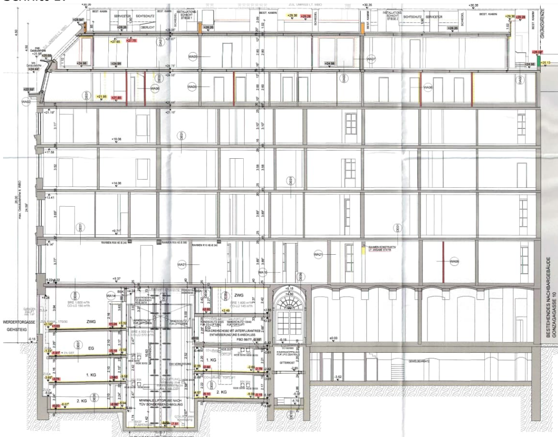
Schnitt 1:
