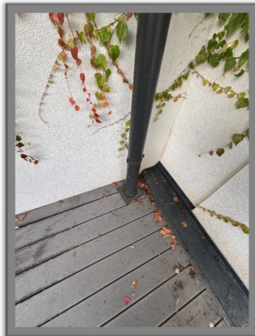
Foto 53: Terrassendetail Reihenhaus
