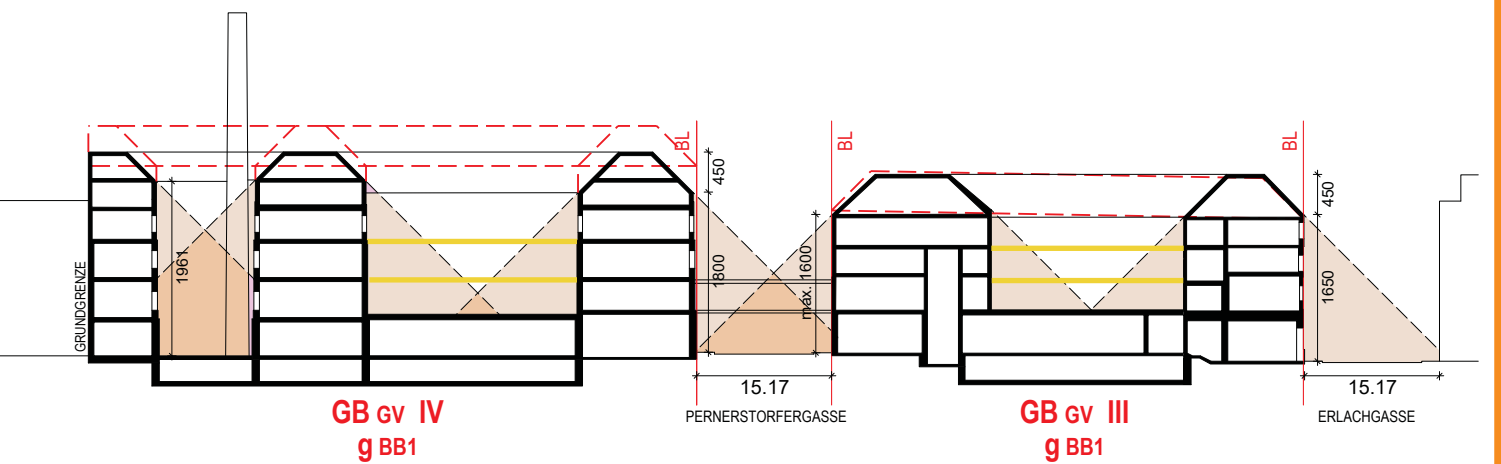
Schnitt / NEU - mit max. Umriss lt. neuen Bauklassen
