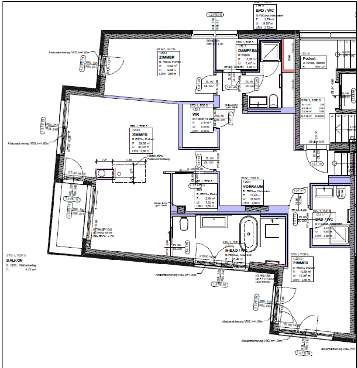
Grundrissplan Top 1.5, 2.OG
