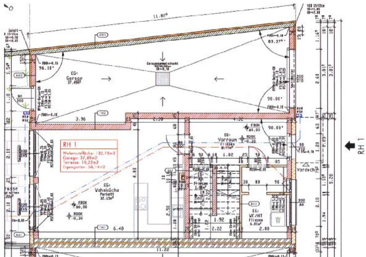
Abbildung 11: Grundriss Erdgeschoß Reihenhause 1 | 21.10.2021
