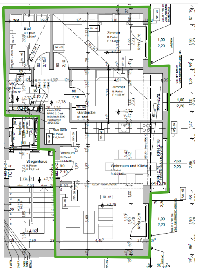
Abbildung 16: Planansicht Wohnung Top 3 Stiege 1 24 , ggst. Wohnung näherungsweise grün markiert
