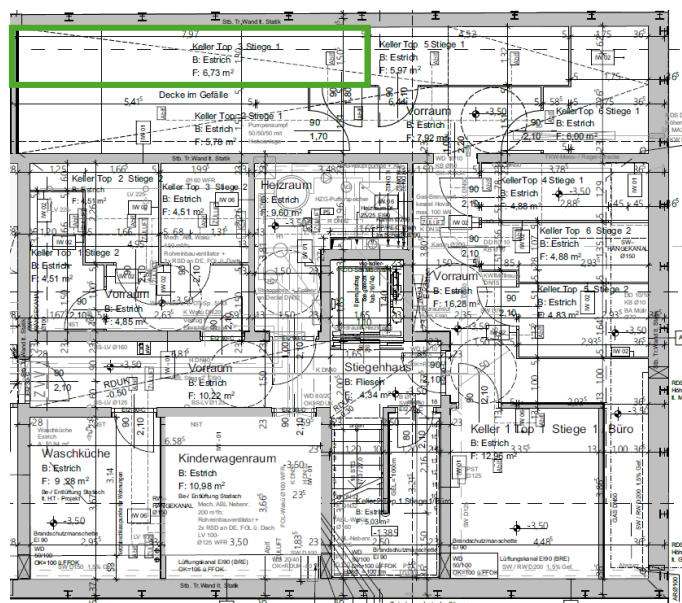
Abbildung 18: Planansicht Zubehör Kellerabteil der Wohnung Top 3 Stiege 1 26 , ggst. Kellerabteil näherungsweise grün markiert
