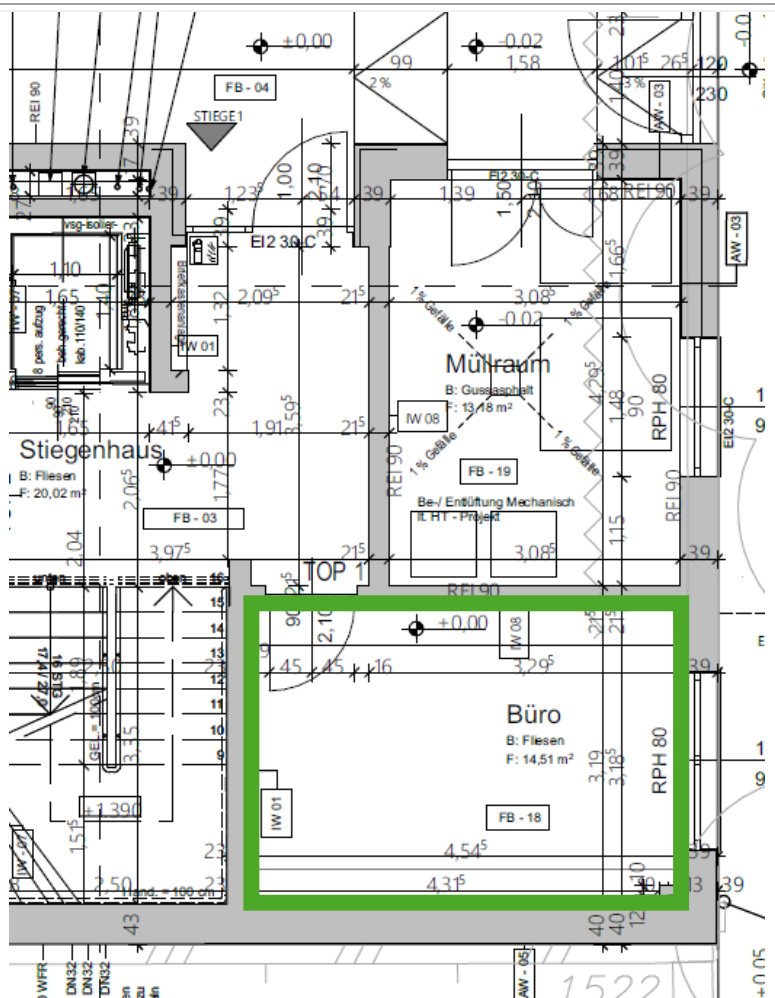
Abbildung 16: Planansicht Büro Top 1 Stiege 1 24 , ggst. Büro näherungsweise grün markiert
