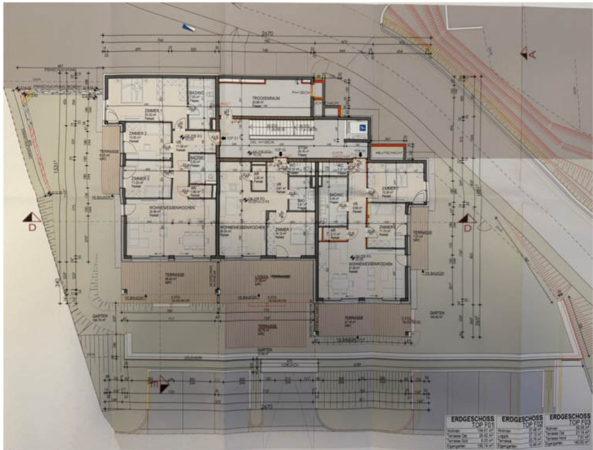
Abb. 33: Grundriss Erdgeschoss Haus F
