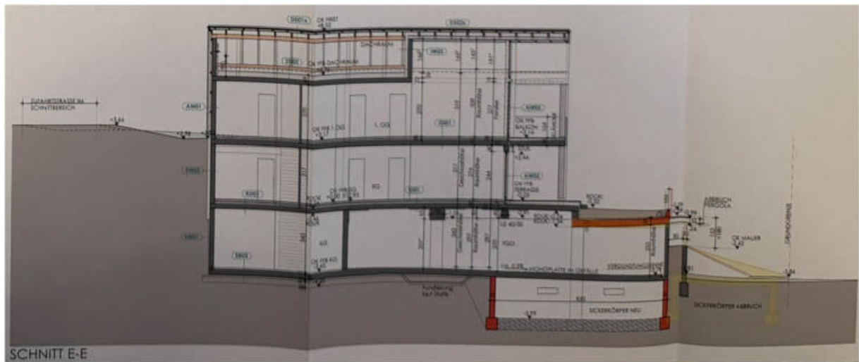
Abb. 31: Schnitt Haus F
