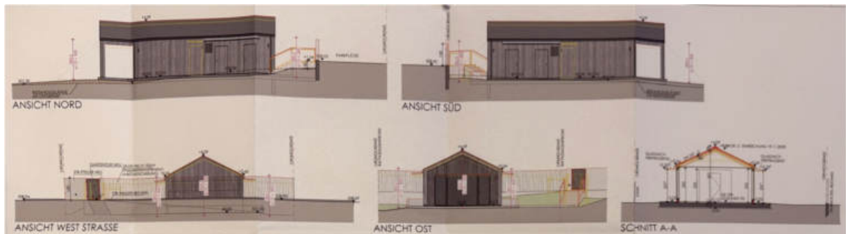
Abb. 20: Pläne Seeparzelle und Badekabinengebäude
