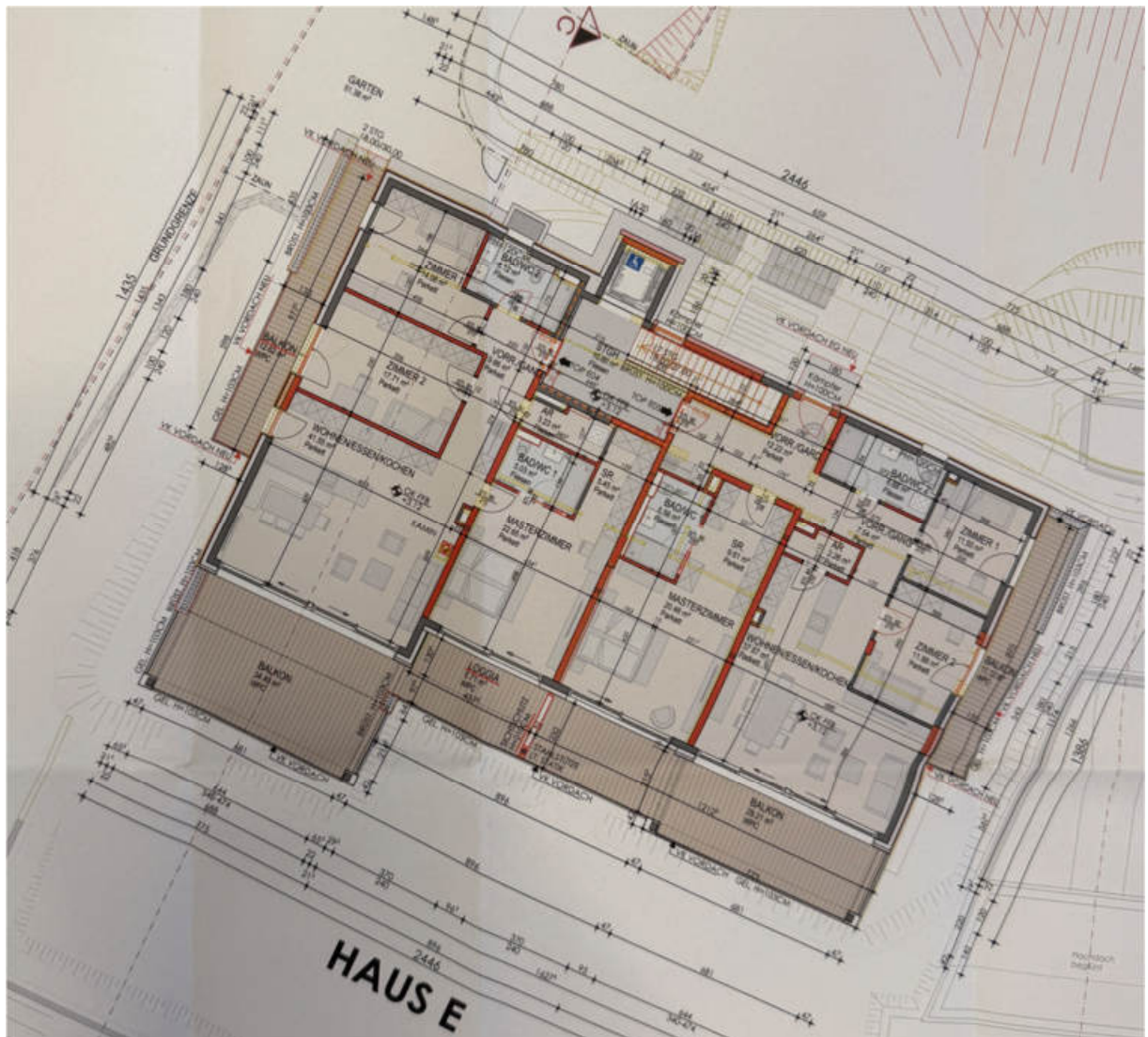
Abb. 32: Grundriss Obergeschoss Haus E
