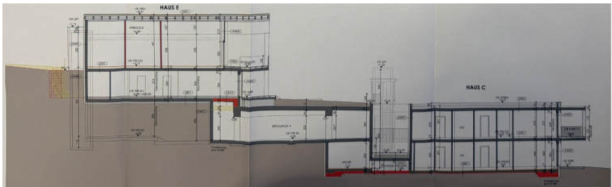
Abb. 31: Schnitt C-C Haus C und Haus E
