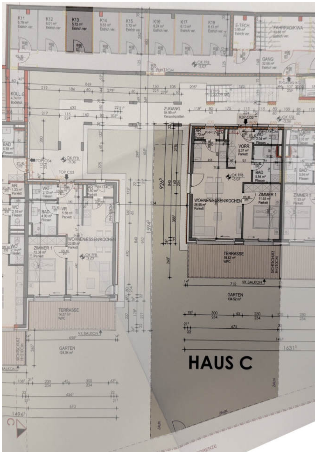
Abb. 35: Wohnung C02 mit Garten C02 und Kellerabteil K13
