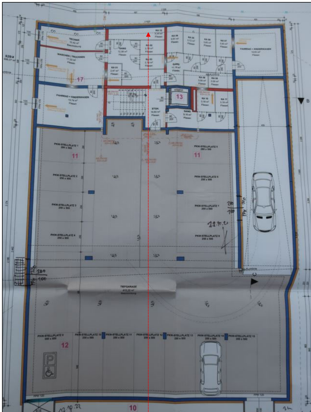
Grundrissplan KG/TG, Kellerabteil 12 (aus baubewilligtem Austauschplan 2022) Kfz-Abstellplätze 6 Top 18, 9 Top 21, 10 Top 22 und 13 Top 25 siehe Beilage 9, Abb. 41 bis 44
