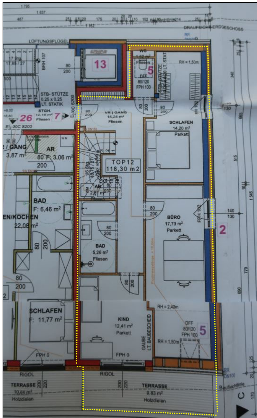
Grundrissplan DG (1. Ebene), Wohnung 12 Top 12 (aus baubewilligtem Austauschplan 2022)
