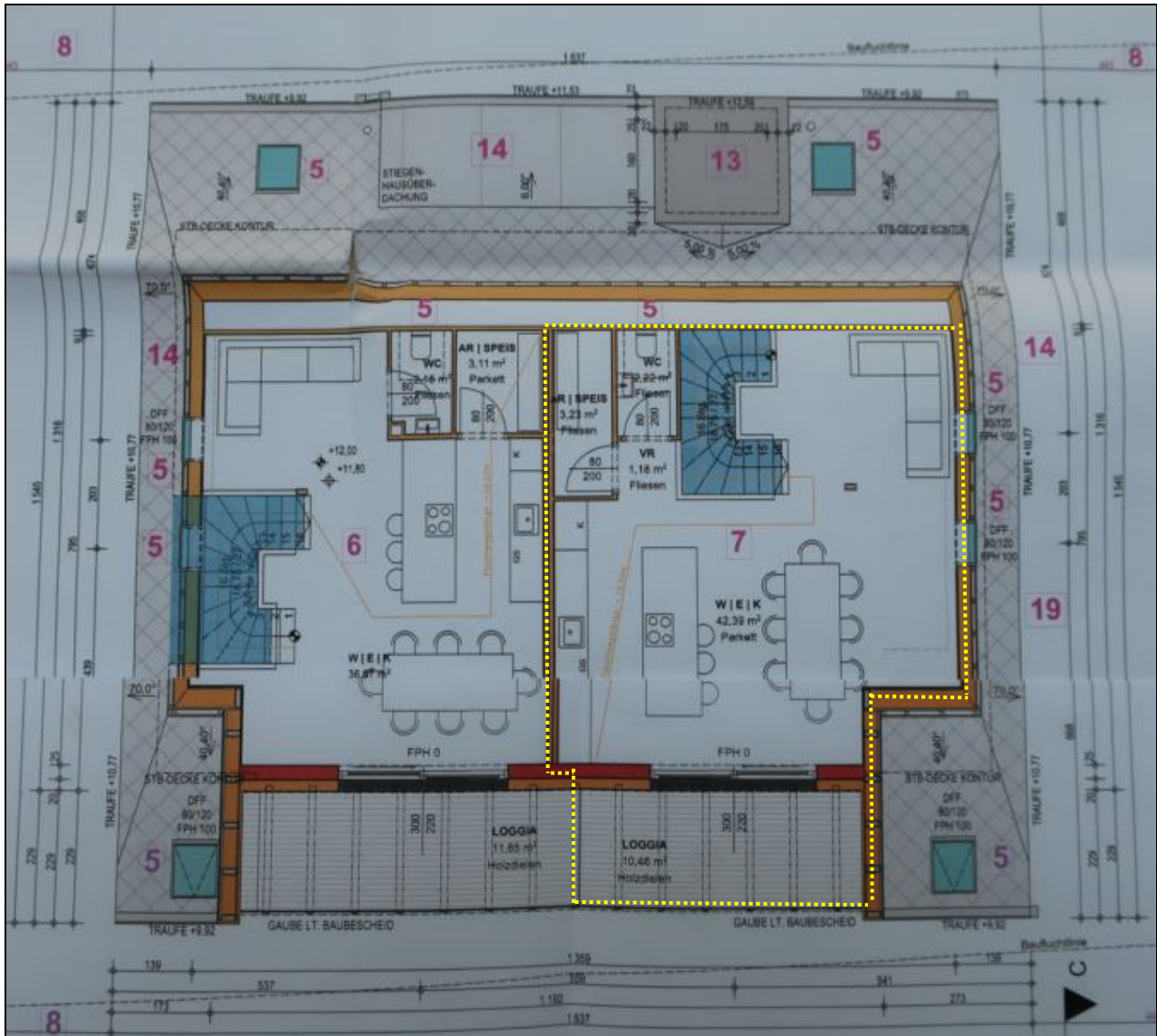
Grundrissplan DG (2. Ebene), Wohnung 12 Top 12 (aus baubewilligtem Austauschplan 2022)
