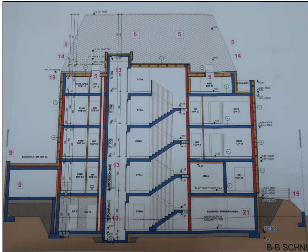
Gebäudeschnitt 1 (aus baubewilligtem Austauschplan 2022)
