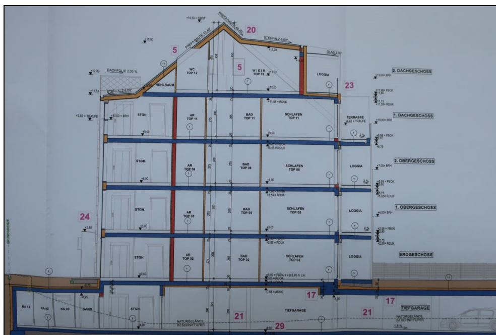
Gebäudeschnitt 2 (aus baubewilligtem Austauschplan 2022)
